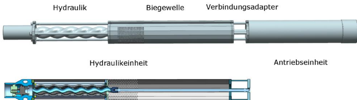
Aufbau einer Exzentrerschneckenpumpe
