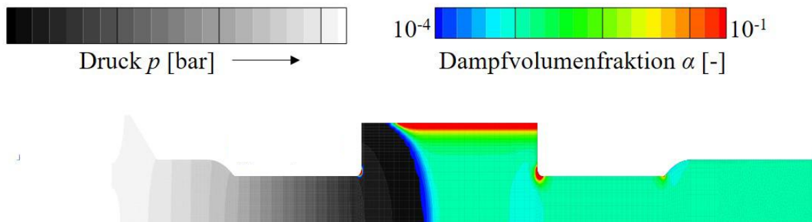
Kavitationsgebiete im Arbeitsraum nach dem Auftreffen einer Druckwelle
